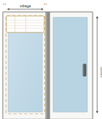
VUE FACE • POSE SUR OUVRANT
