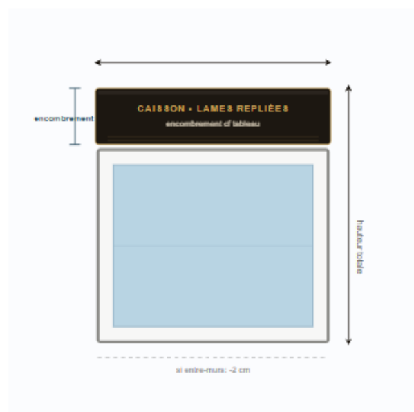
VUE FACE • POSE AU-DESSUS
